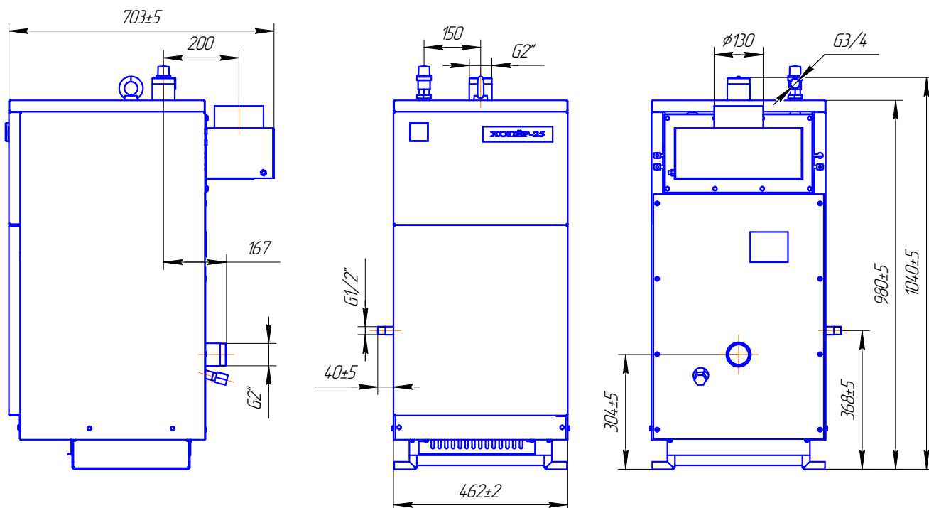
Рис. 1. Габаритные и присоединительные размеры
