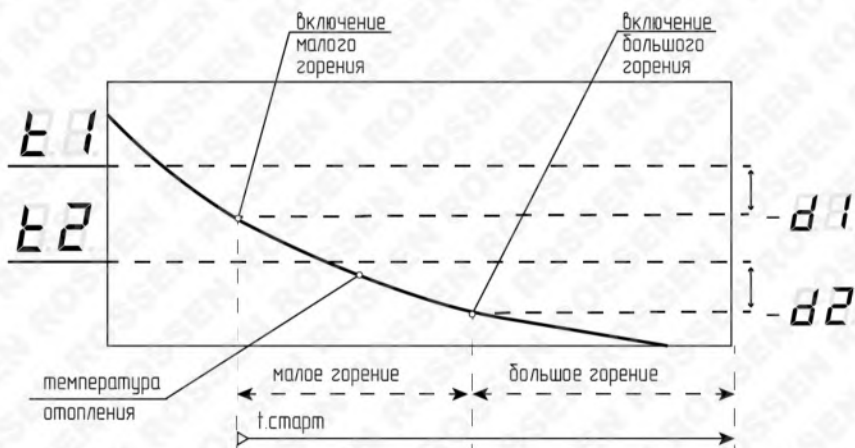
Рисунок 14. Динамика работы котла при охлаждении.
