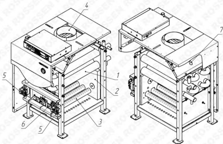
1 - оребренная труба теплообменника, 2 – теплоизоляция топки, 3 - рожек горелки, 4 - выход дымовых газов (газоход), 5 - газовый клапан, 6 - датчик тяги, 7 - отверстие для замера параметров отходящего газа.
