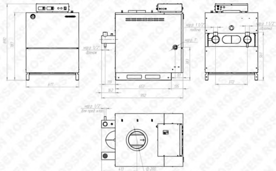
Рисунок 1. Габаритно-присоединительные размеры котла RSA40, RSA60
