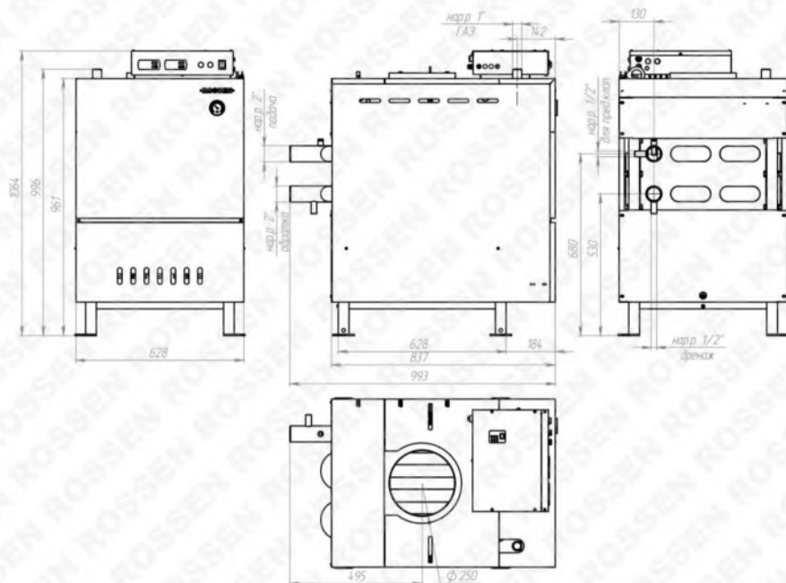
Рисунок 3. Габаритно-присоединительные размеры котла RSA100
