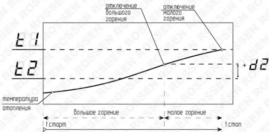
Рисунок 13. Динамика работы котла при нагреве.
