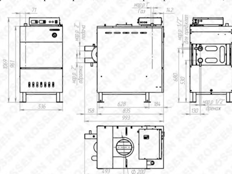
Рисунок 2. Габаритно-присоединительные размеры котла RSA80
