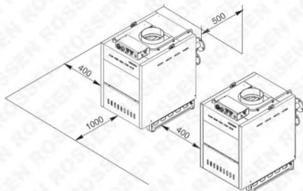
Рисунок 20. Минимальные расстояния до котла.
