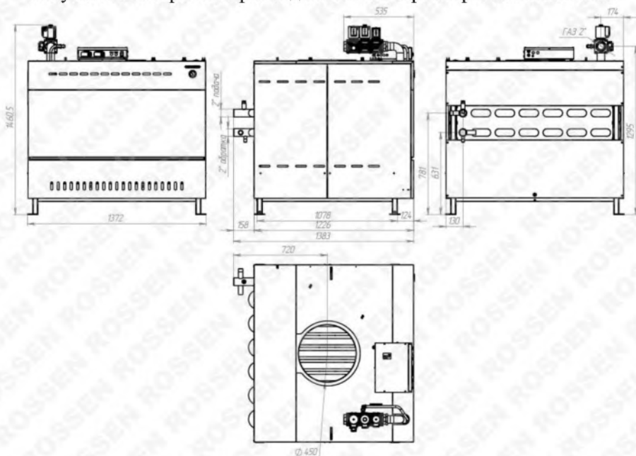
Рисунок 4. Габаритно-присоединительные размеры котла RSA500
