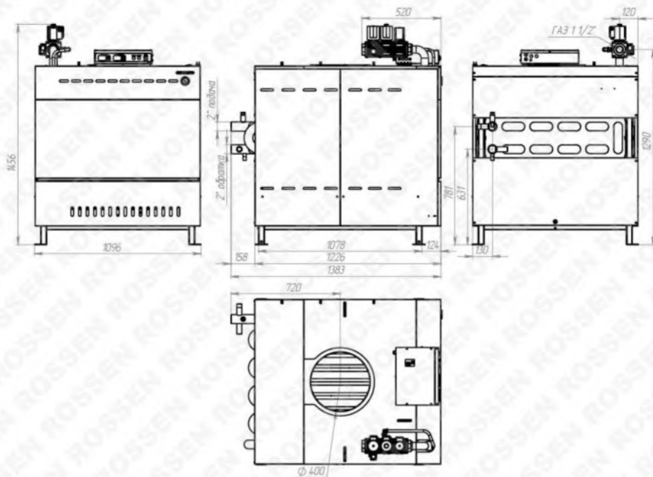
Рисунок 3. Габаритно-присоединительные размеры котла RSA400
