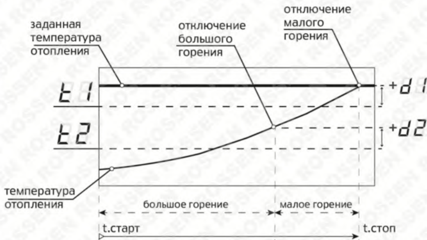
Рисунок 14. Динамика работы котла при нагреве.
