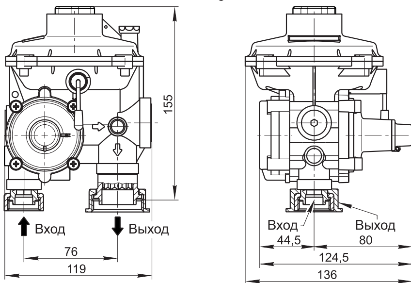
Исполнение - П-образное
