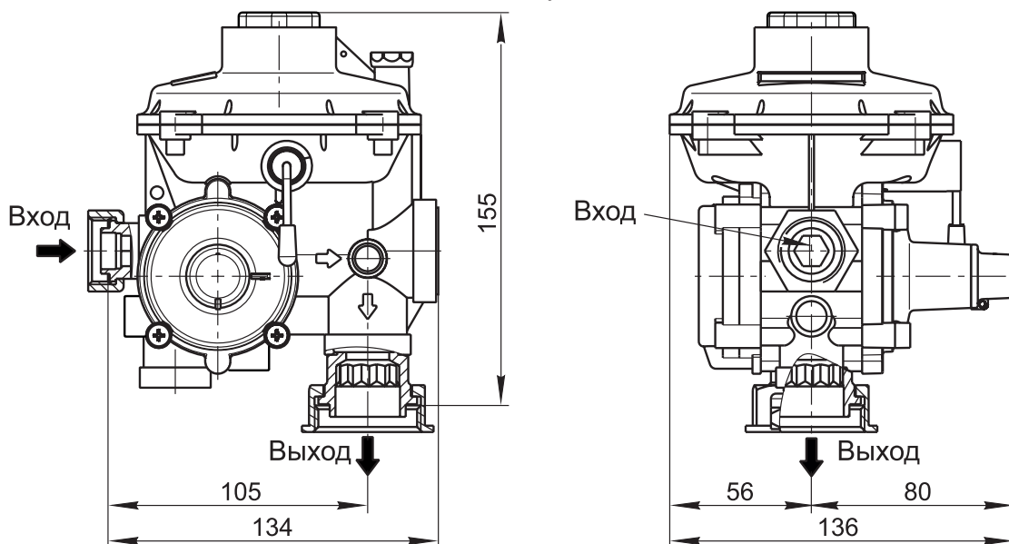
Исполнение - угловое
