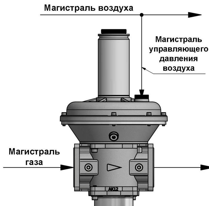
Рис. 12-33. Подсоединение регулятора соотношения давлений газ-воздух (исполнение 1)
