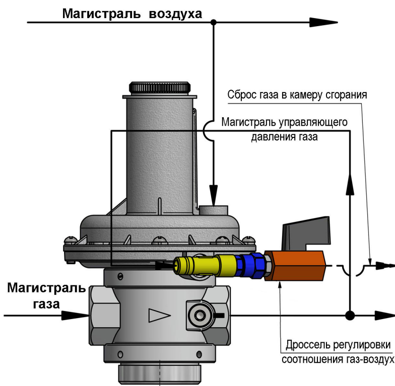
Рис. 12-35. Комплект регулятора соотношения давлений газ-воздух и дроссельного узла, устанавливаемого на газовую магистраль (исполнение 3)
