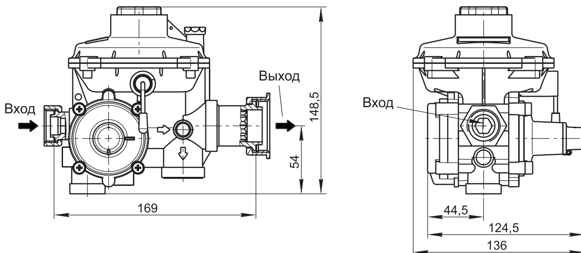
Исполнение - линейное
