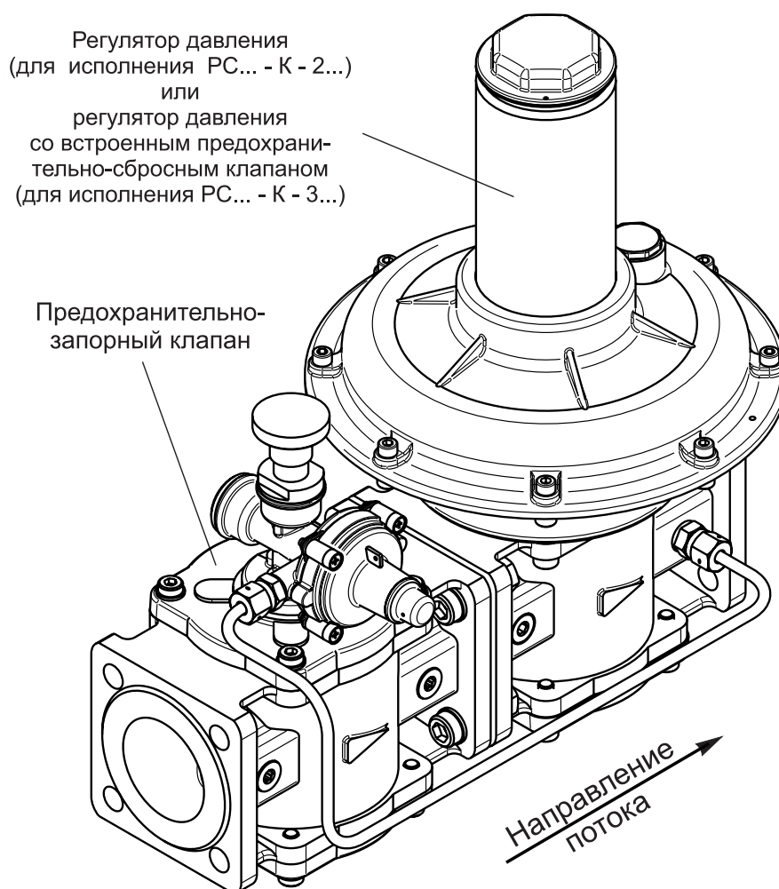
Рис. 12-21. Регуляторы-стабилизаторы давления с предохранительно-запорным клапаном (исполнения РС... - К - 2..., РС... - К - 3...)
